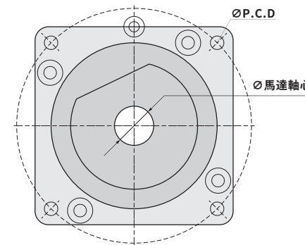
馬達法蘭示意圖 Instruction of Motor Flange
