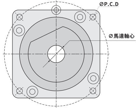
馬達法蘭示意圖
